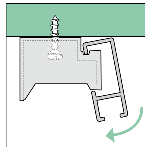
Deckenmontage mit Deckenhaltern / Ceiling mounting with ceiling brackets
