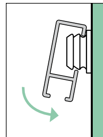
Wandmontage mit Wandklammern / Wall mounting with wall brackets
