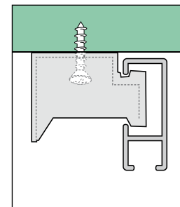
Deckenmontage mit Deckenhaltern / Ceiling mounting with ceiling brackets
